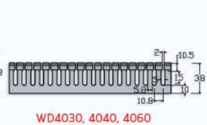
WD4030, 4040, 4060
