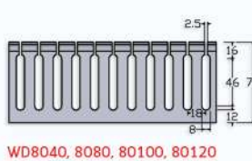
WD8040, 8080, 80100, 80120
