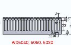
WD6040, 6060, 6080
