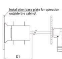
ก้านโยกโยสหน้าตู้ รุ่น 125-1600
